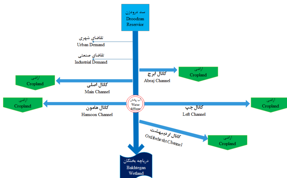
شکل ۱- نمای شماتیک موقعیت کانال های شبکه آبیاری و زهکشی دشت رامجرد در پایین دست سد درودزن
